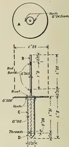
From A. S. T. M. Proc. FIG. 160.—Hubbard's Consistency Tester.
